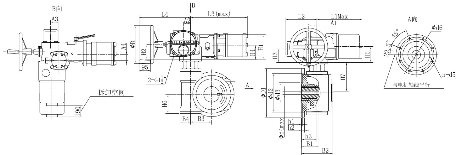
SMC-00~2带HBC外形及连接尺寸
